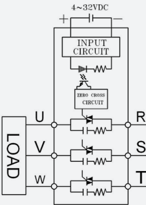
TSR-25DA-□ / TSR-40DA-□
