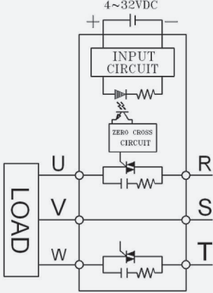
TSR-50DA-□ / TSR-75DA-□
